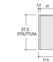
Terminale a giorno con ripiani stondati / Open terminal with shaped shelves
