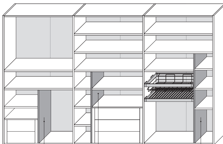
Tramezza / Int. side H. 93
