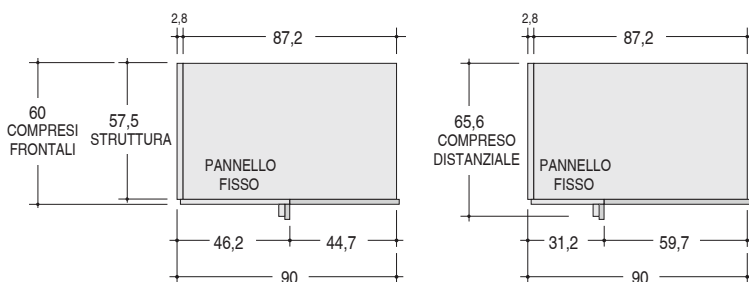
Angolo con pannello fisso e compensatore / Corner with fixed panel and compensator
