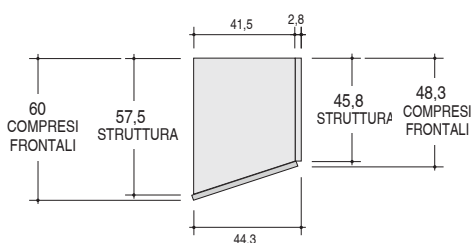
Terminale obliquo / Oblique terminal
